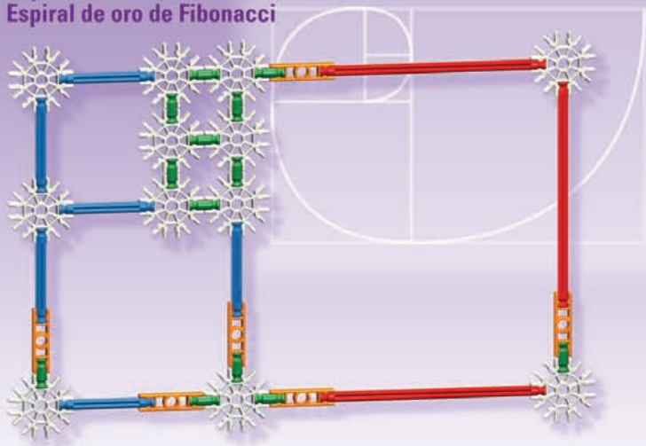
Fibonacci Golden Spiral Spirale d'or de Fibonacci Espiral de oro de Fibonacci
